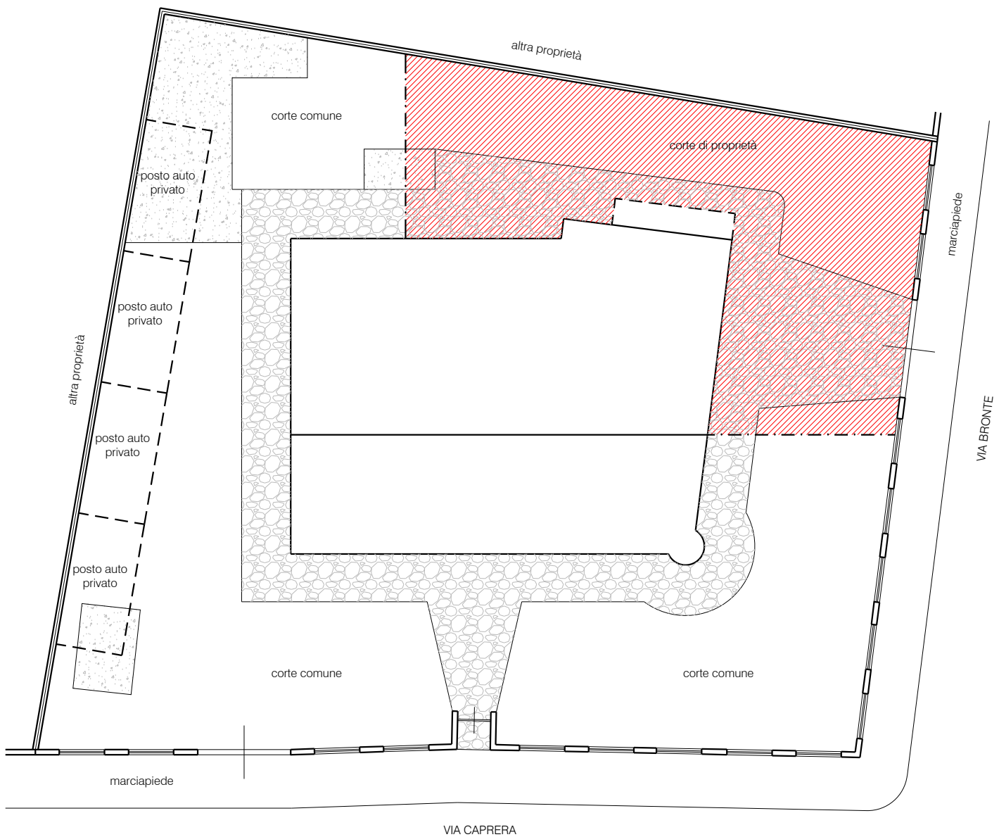
PLANIMETRIA scala 1:200
